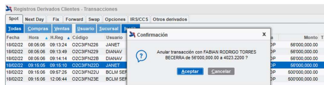
Ilustración 35 Anulación Registro
