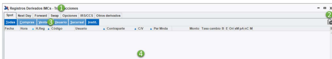
Ilustración 8 Ventana Transacciones
