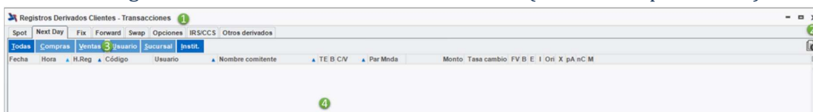
Ilustración 17 Ventana Transacciones
