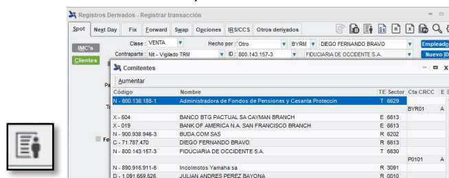
Ilustración 37 Botón Comitentes
